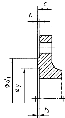
Form F: Rücksprung
