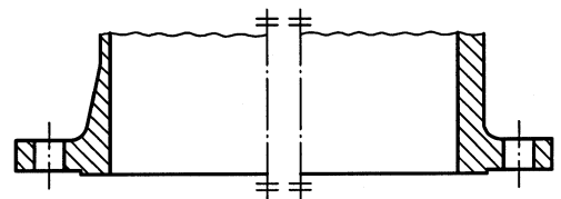
Typ 21 Integralflansch
