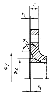
Form F: Rücksprung
