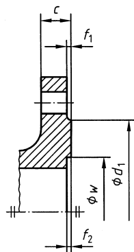
Form E: Vorsprung
